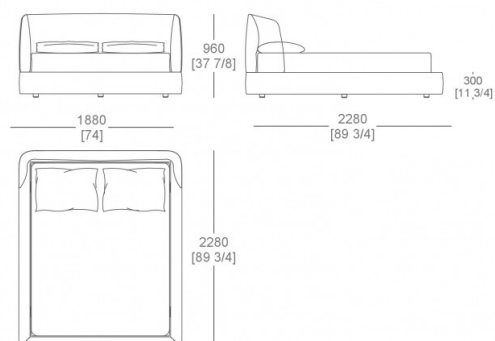
Letto rete alzabile (materasso L. 1800 x P. 2000 mm)
