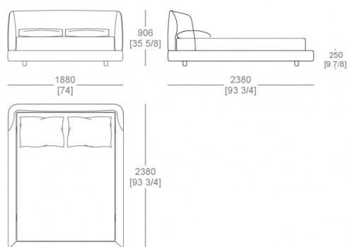
Letto rete fissa (materasso L. 1600 x P. 2100 mm)
