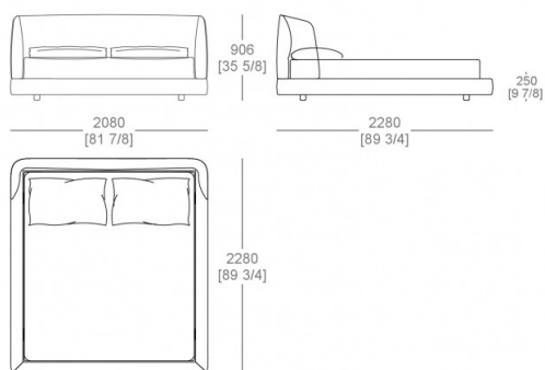
Letto rete fissa (materasso L. 1800 x P. 2000 mm)
