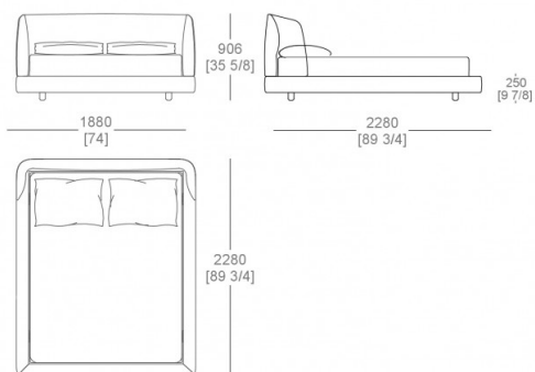
Letto rete fissa (materasso L. 1600 x P. 2000 mm)
